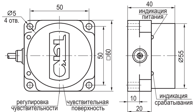
Габаритный чертеж
